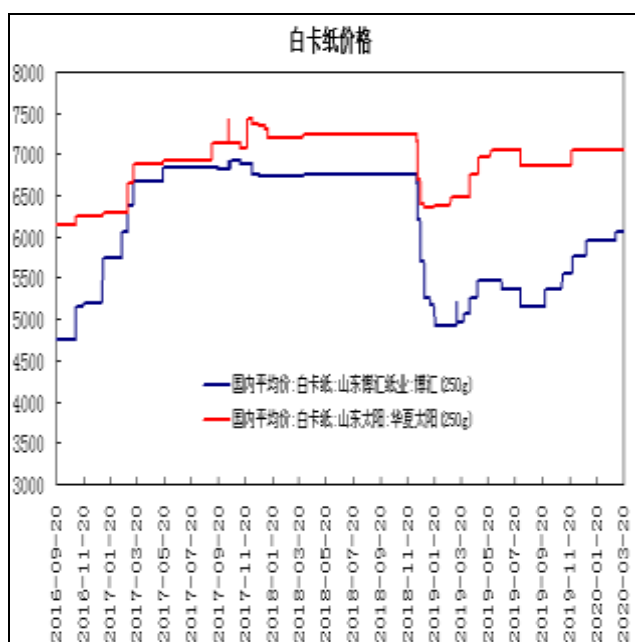
图17：白卡纸价格
