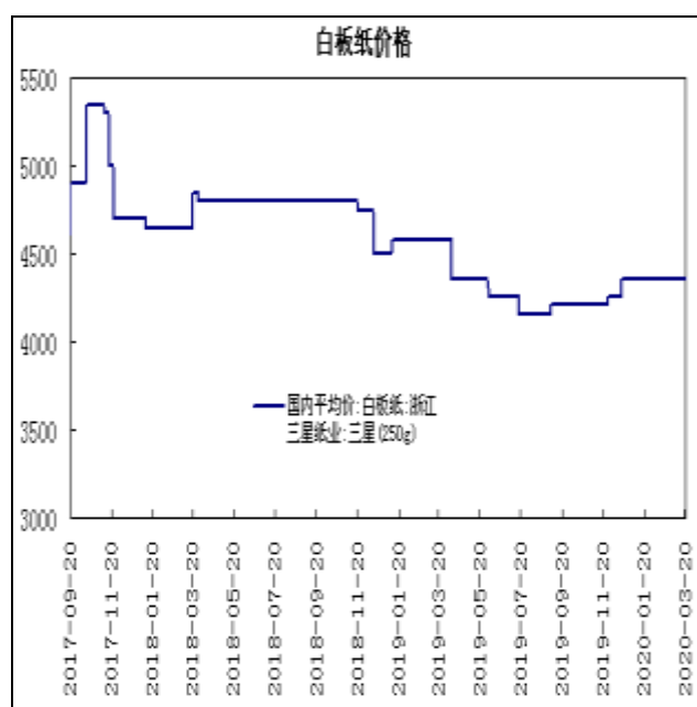
图18：白板纸价格
