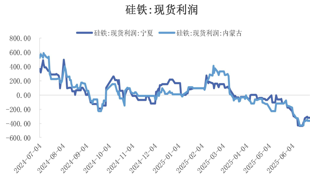
图14、硅铁现货生产利润 单位：元/吨
