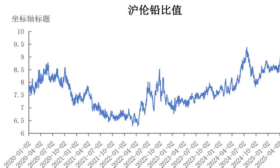
图2 沪伦比值
