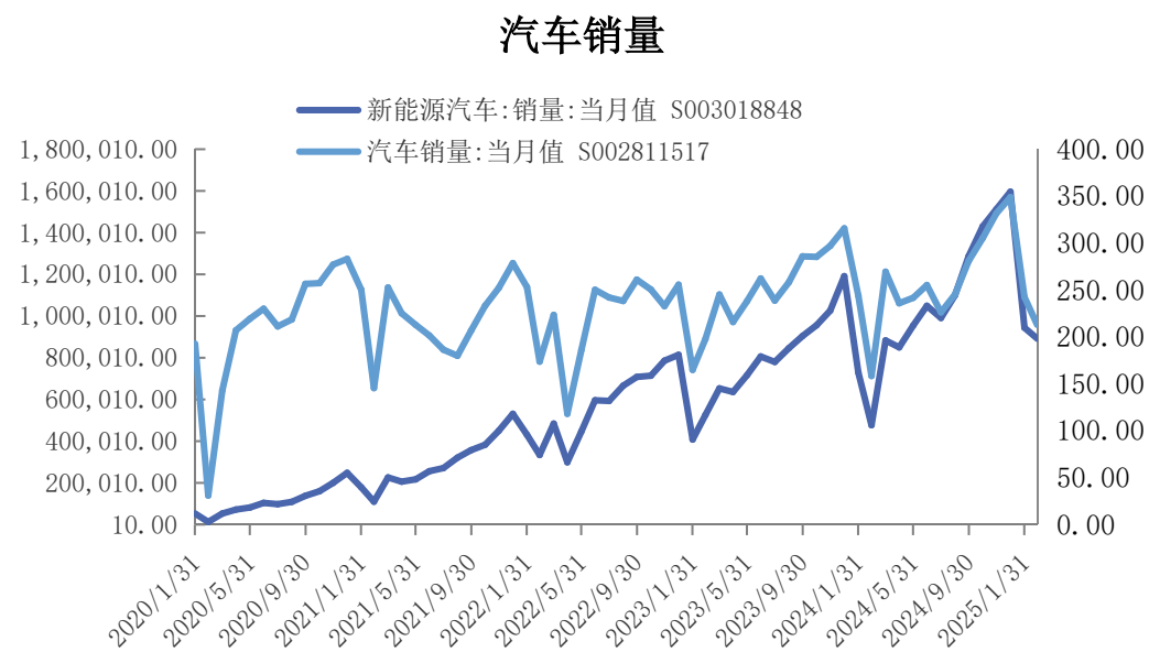
图16 汽车产销
