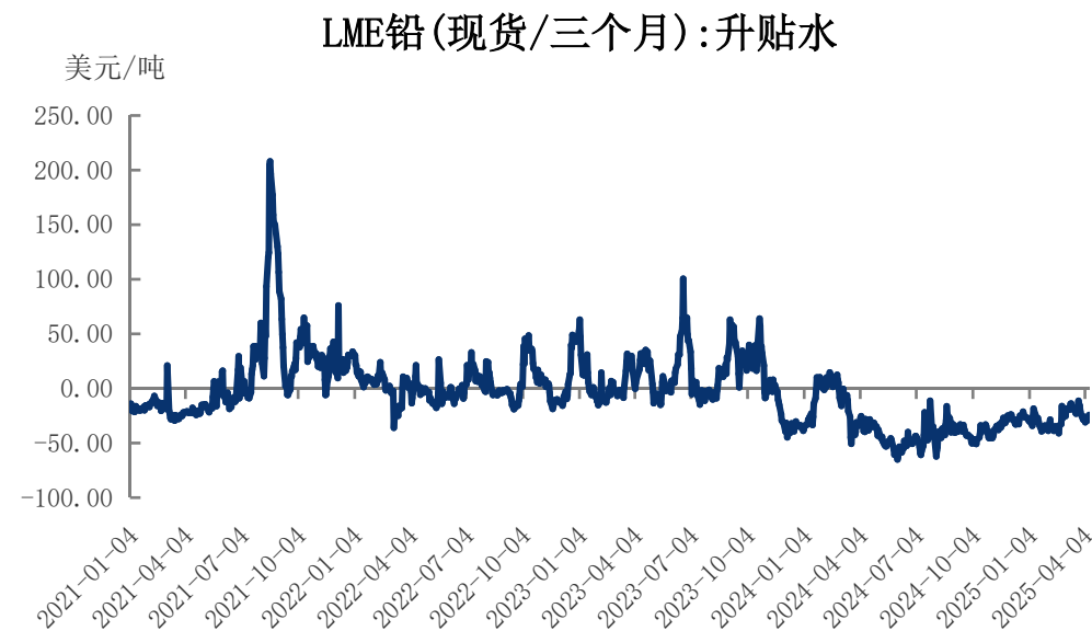
图5 LME升贴水
