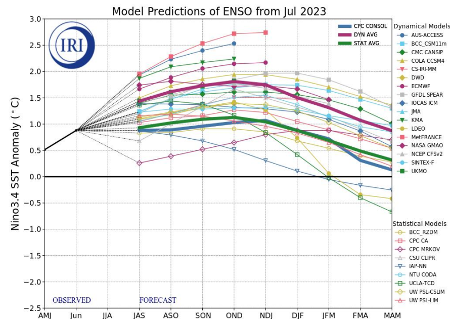
图 不同模型对ENSO指数的预测（7月）
