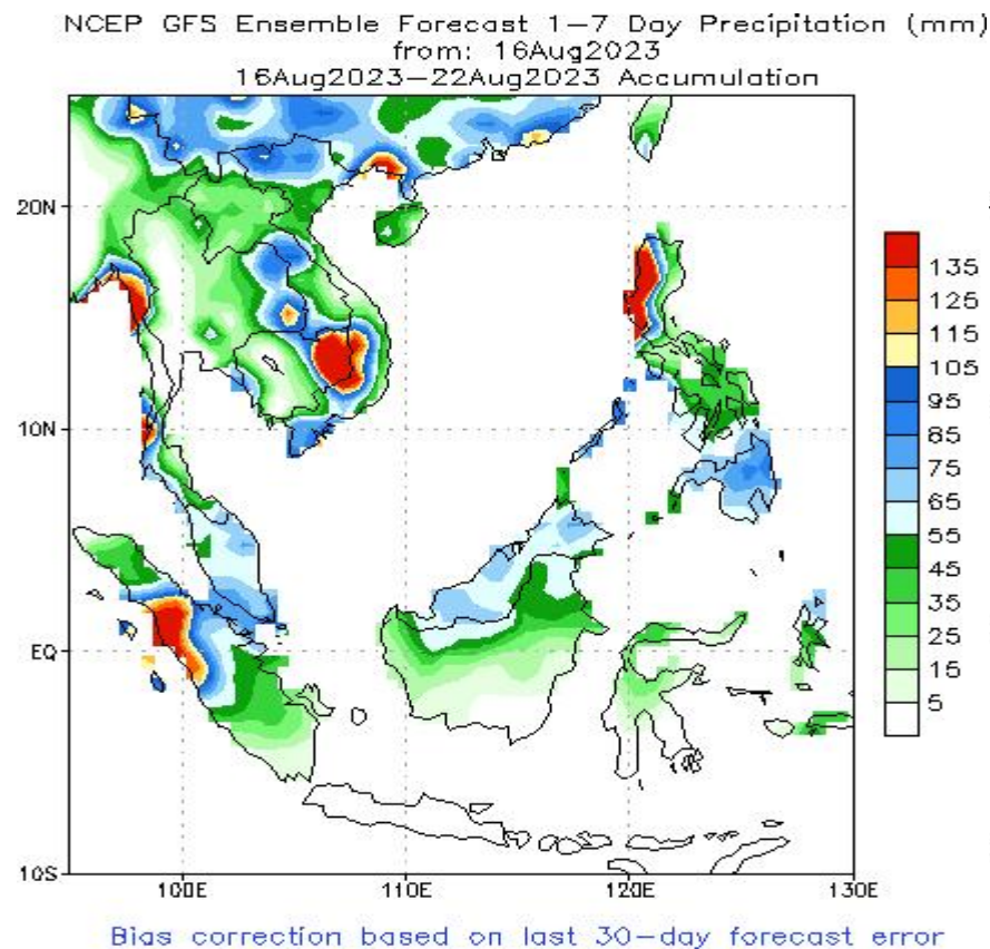
图 东南亚未来一周降水
