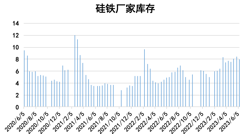
图10、硅铁库存
