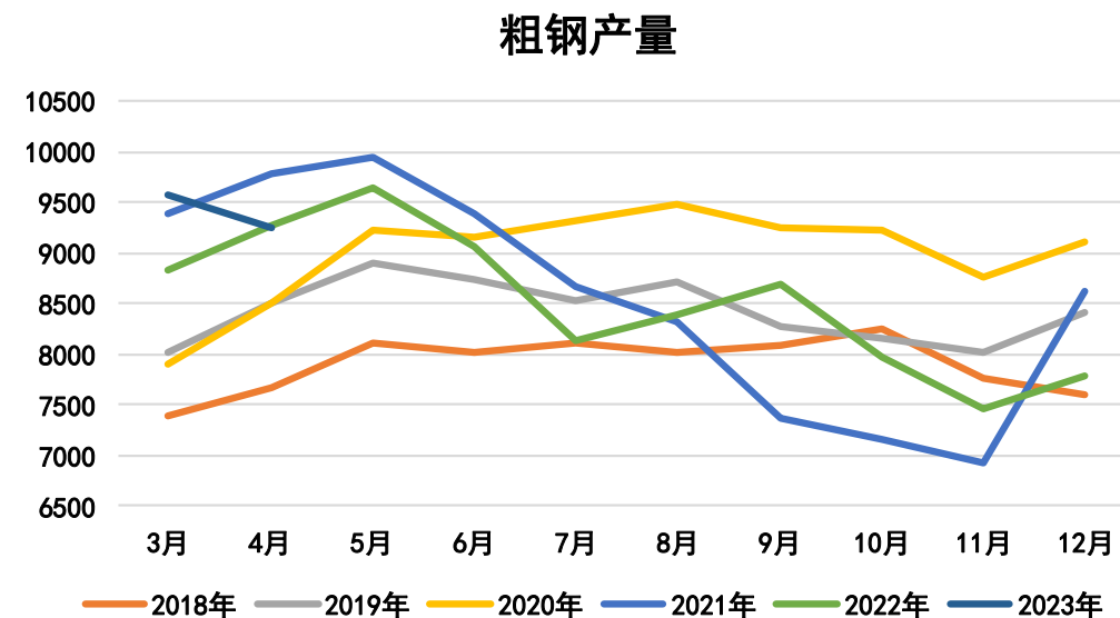
图15、粗钢产量
