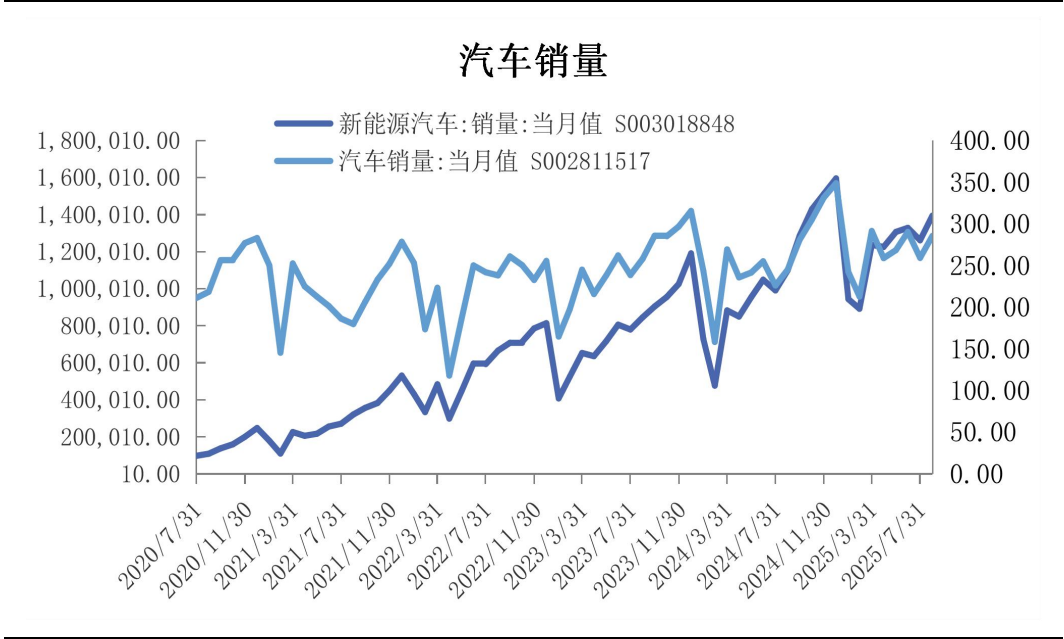
图16 汽车产销
