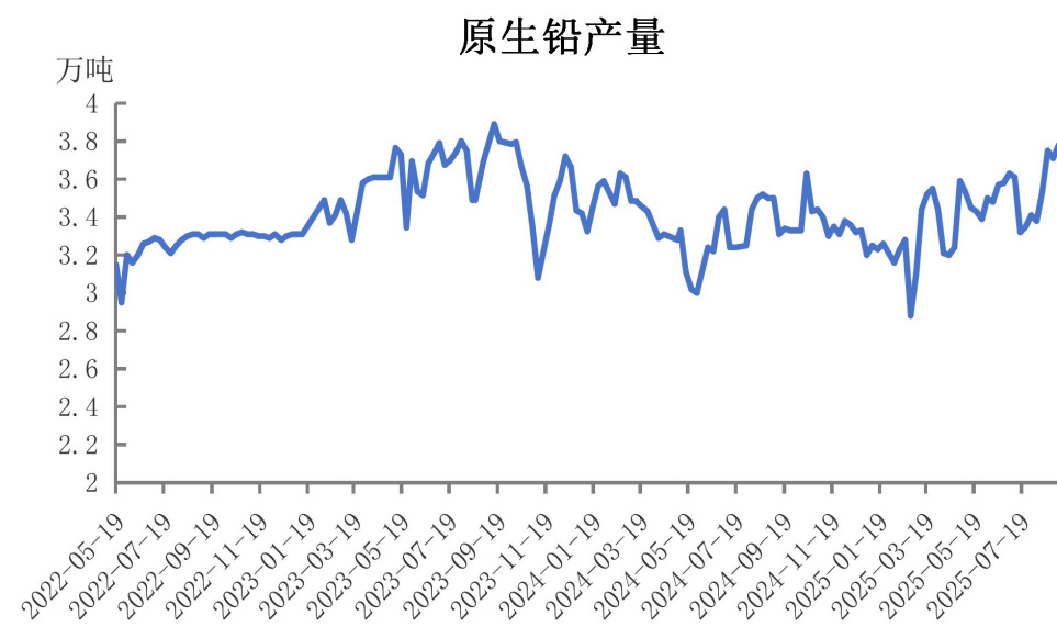
图7 原生铅产量
