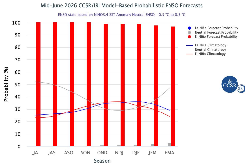
图 ENSO预测（6月）
