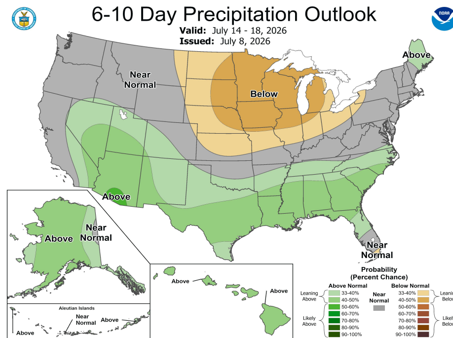
图 降水量前瞻
