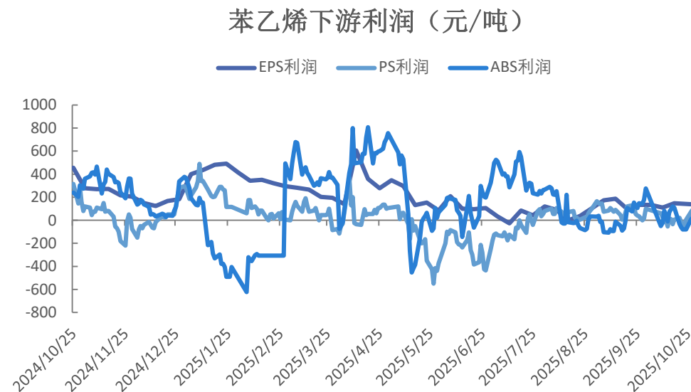
图22、EPS、PS、ABS利润
