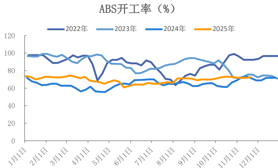
图18、ABS开工率
