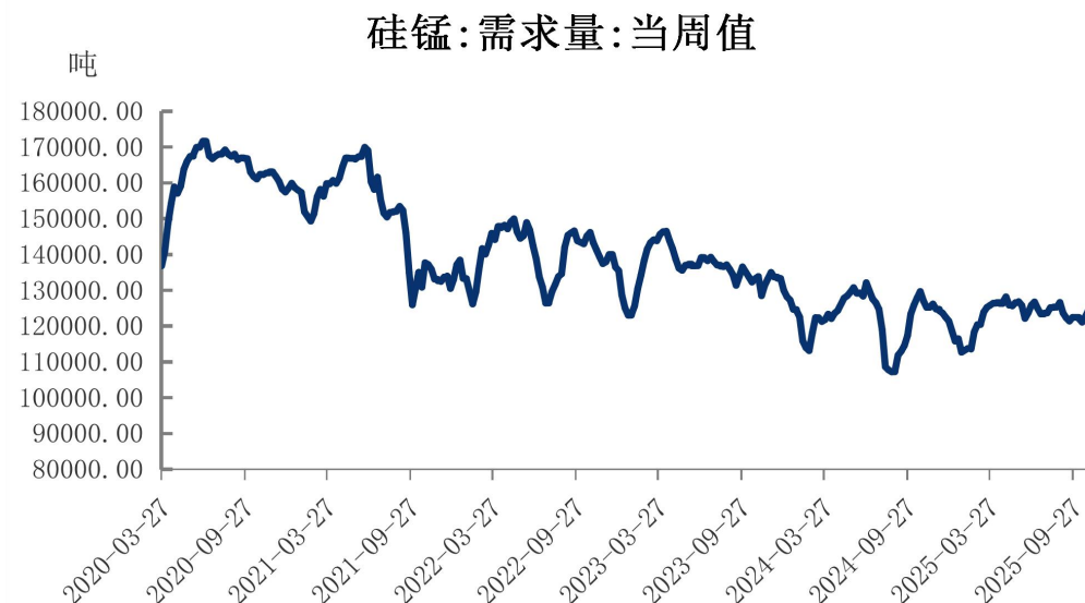
图8、硅锰需求量当周值
