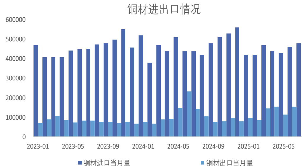
图22、铜材进出口
