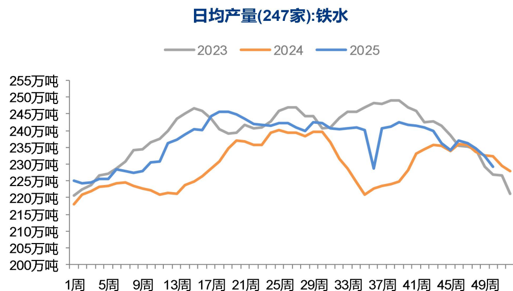
图15、铁水产量
