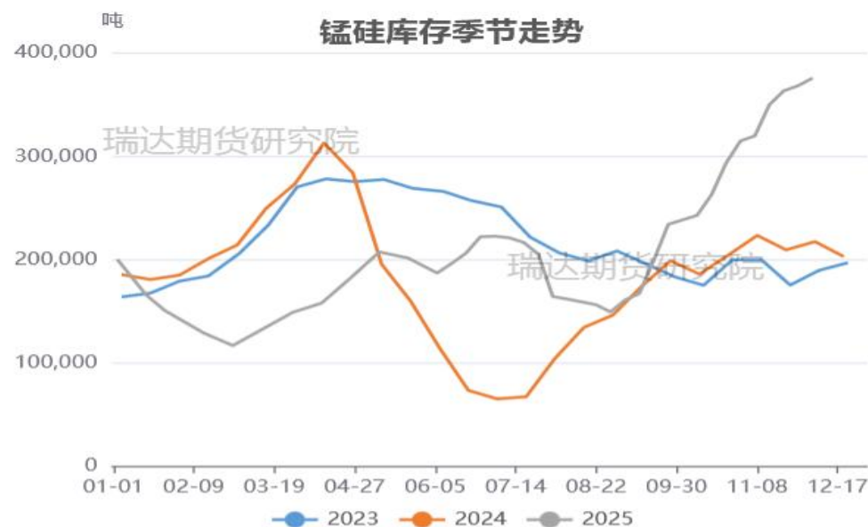
图9、硅锰库存
